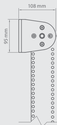
Rozměry nástěnno-stropního držáku
