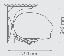
Stropní montáž
