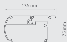
Przekrój belki przedniej
