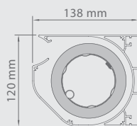
Průřez kazety
