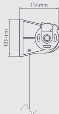
Wymiary uchwytu ścienna-sufitowego
