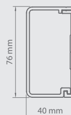
Przekrój prowadnicy
