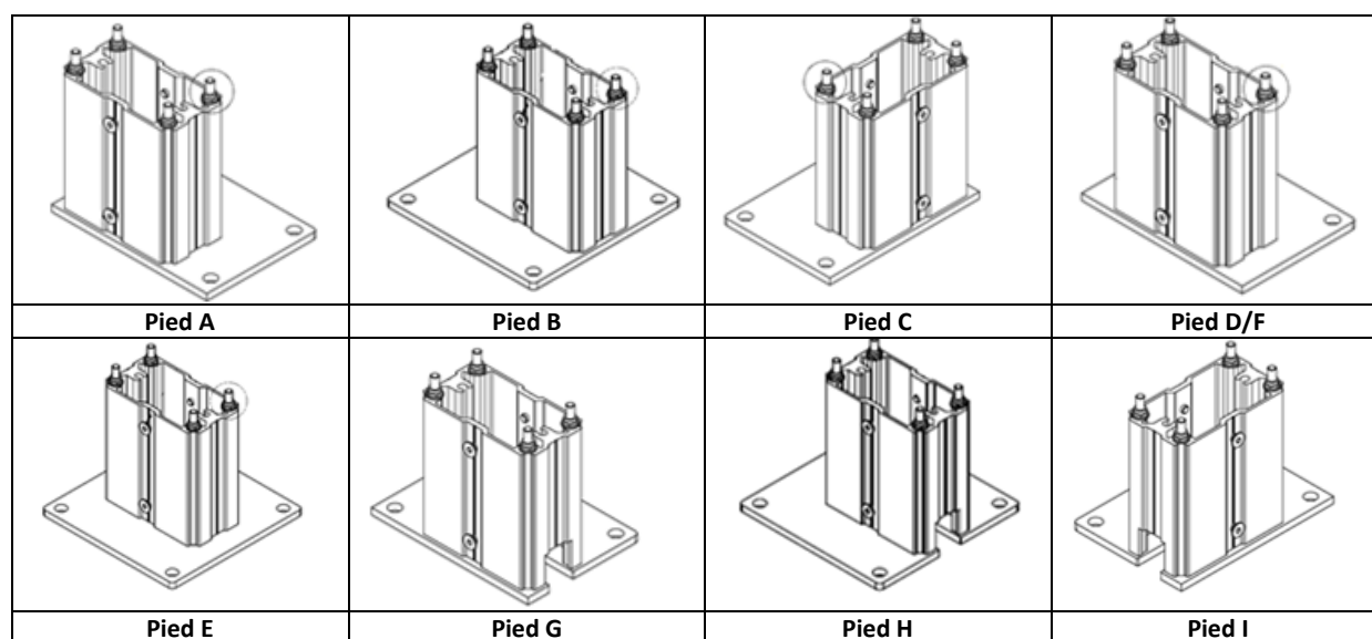
Fig. 7. Types des pieds de la pergola SB400
