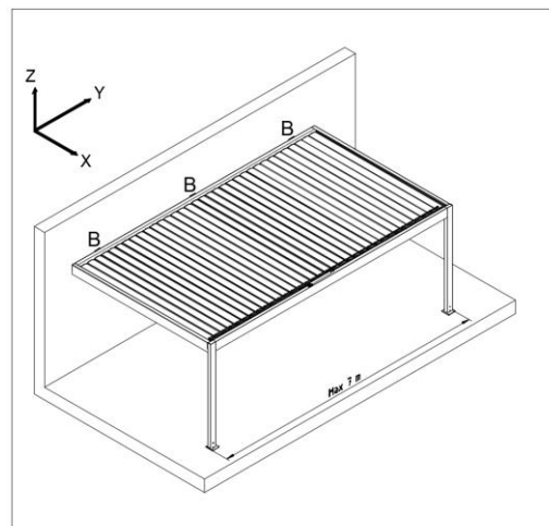
B – Support mural monté à la barre.
