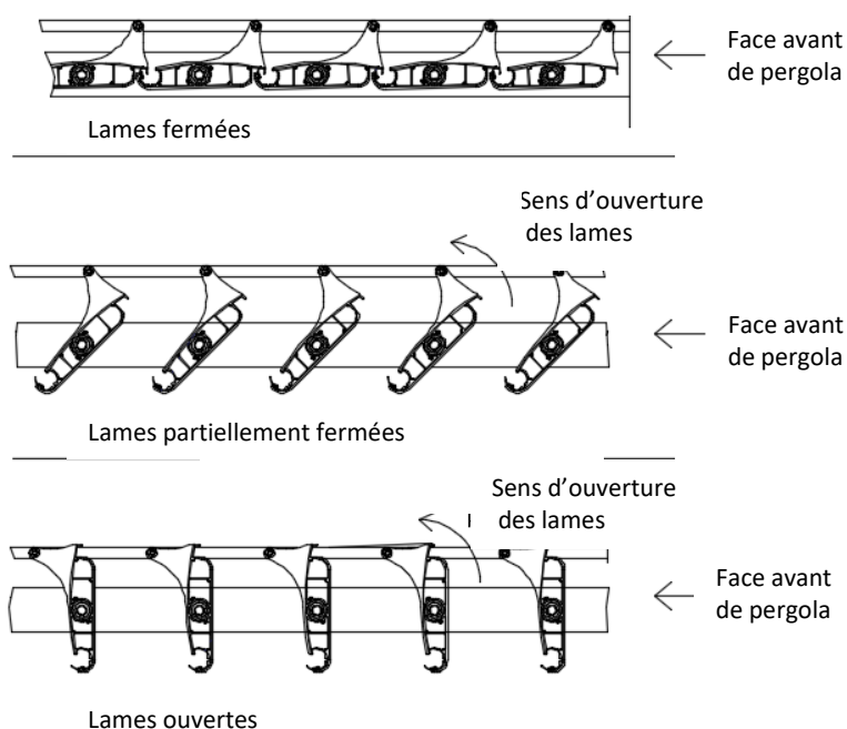
Fig. 3 Réglage standard du sens d'ouverture des lames pour la Pergola SB400
