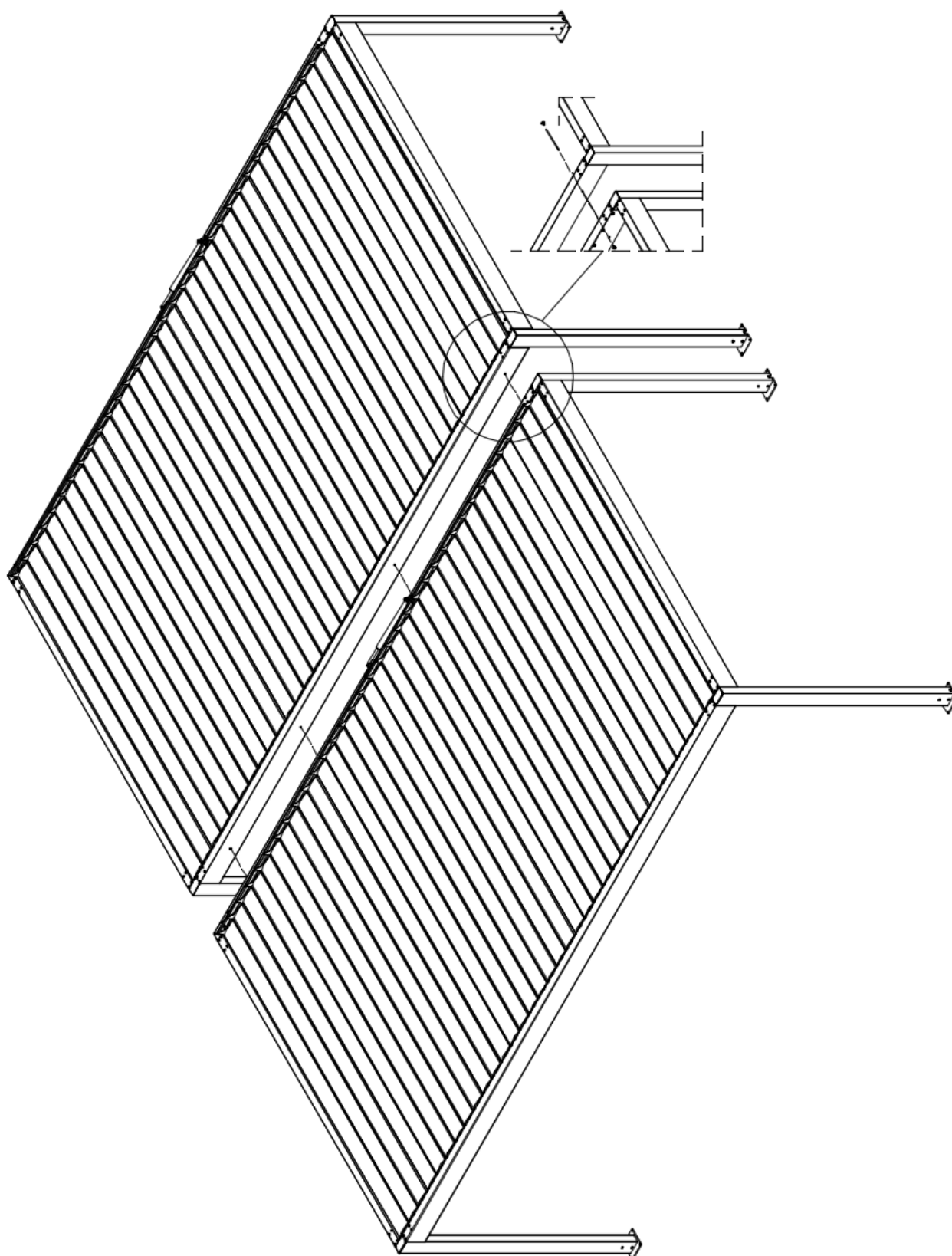
Fig. 5. Vue de l'assemblage des modules de la Pergola SB 400
