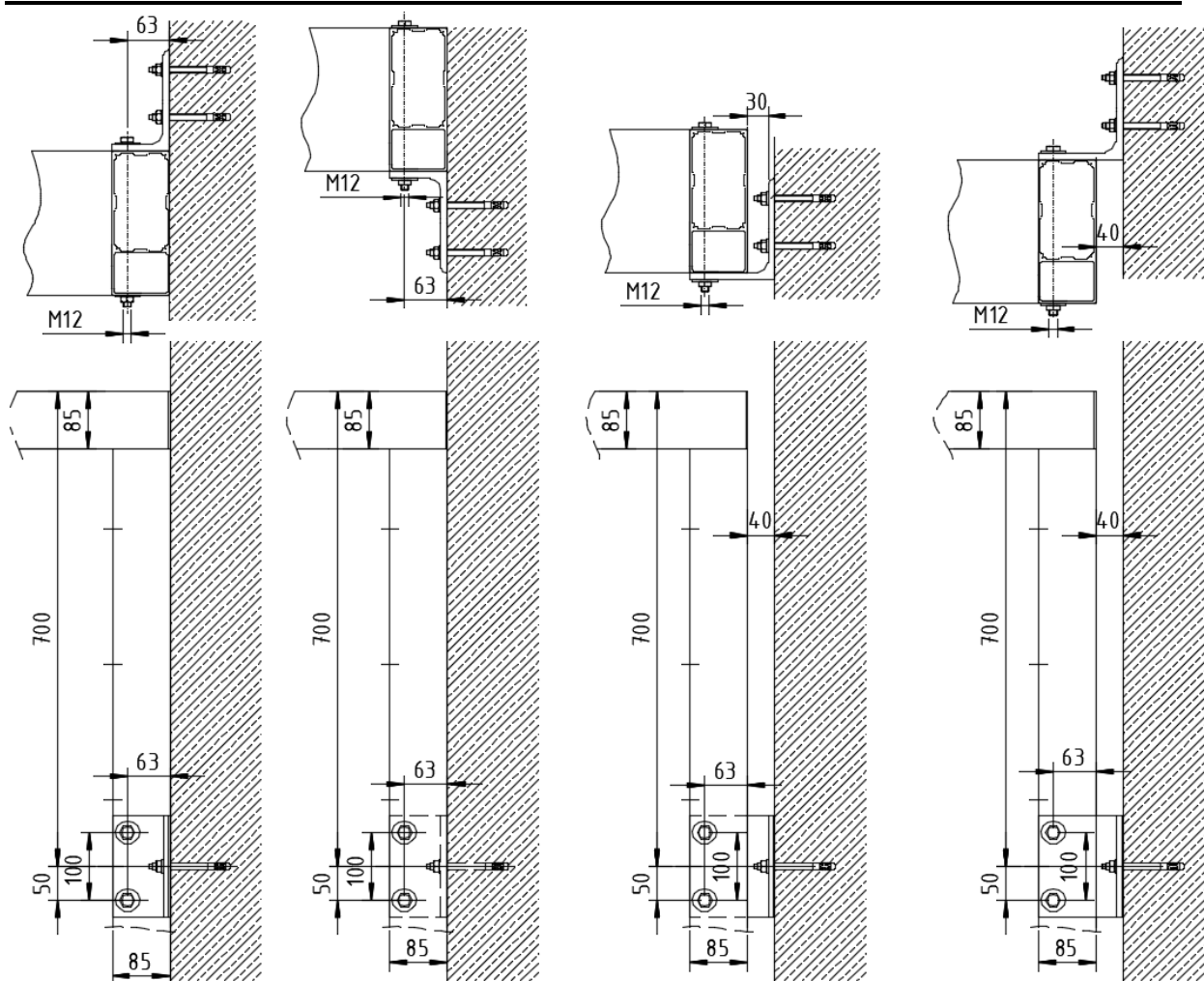
Version murale courte (vue de côté et vue de dessus)
