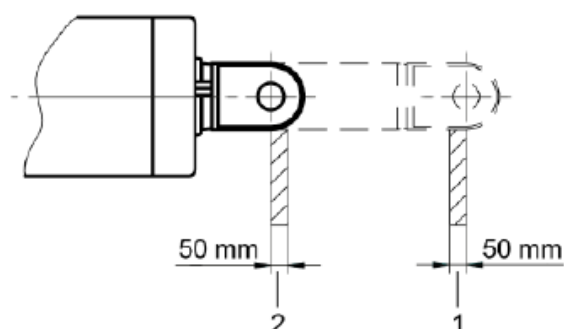
Figure 30 La réduction des courses du moteur admissible.
