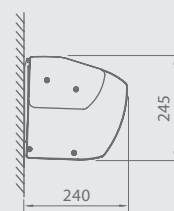
Fixation au mur
