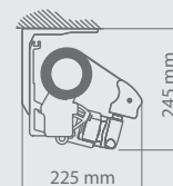
Fixation au plafond
