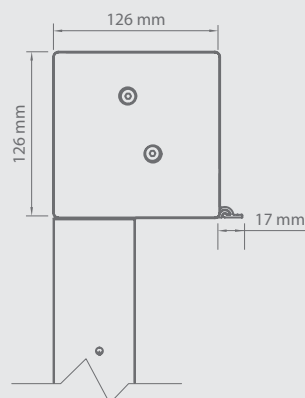
Dimensions de caisson
