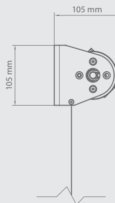
Dimensions des supports muraux et de plafond
