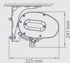
Fixation au plafond
