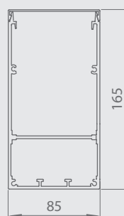
Profil de la barre
