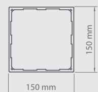
Section du poteau
